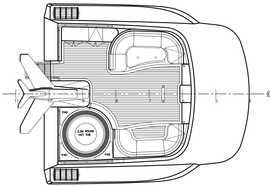
FLYBRIDGE
